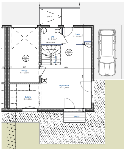
REZ-DE-CHAUSSEE
