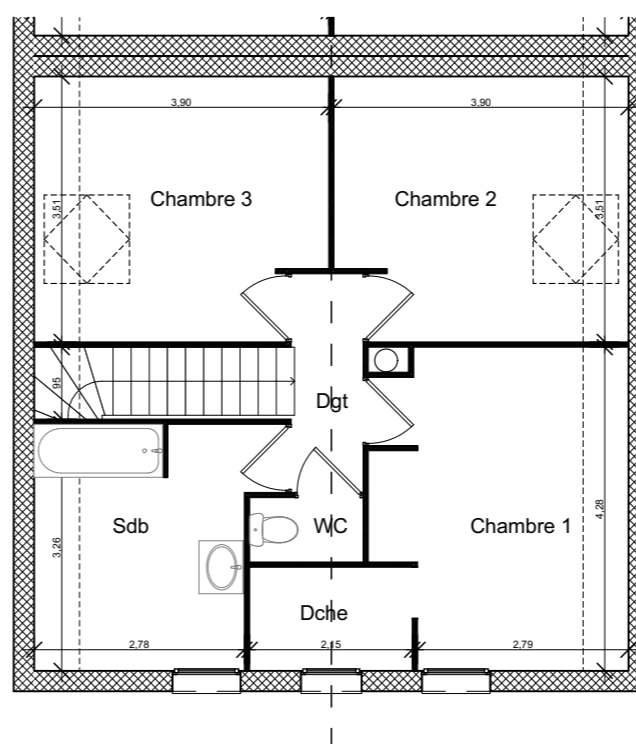
ETAGE
