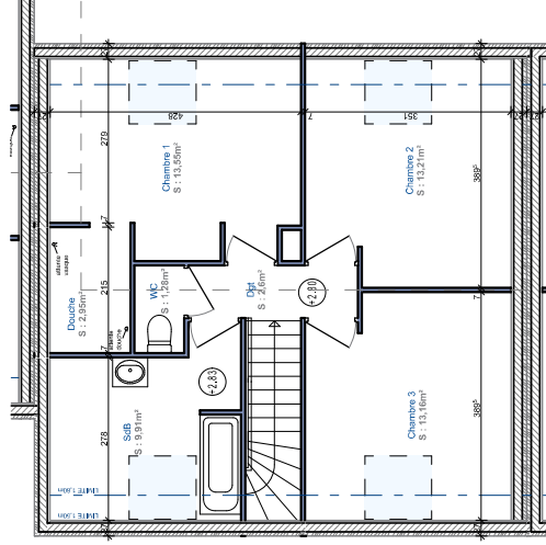
ETAGE
