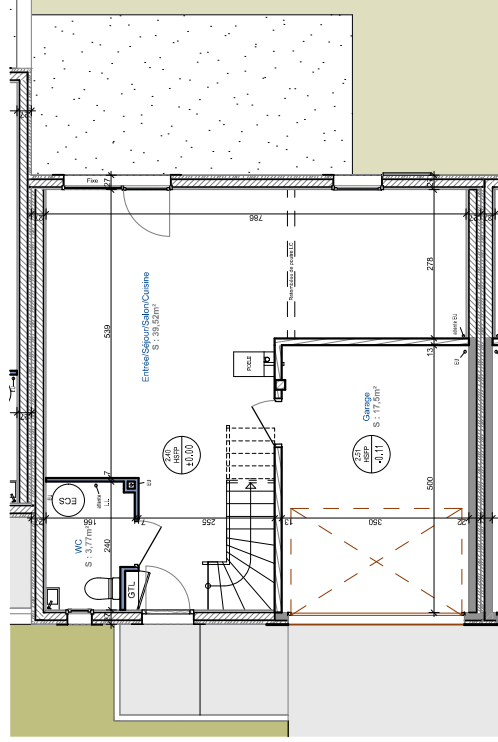
REZ-DE-CHAUSSEE
