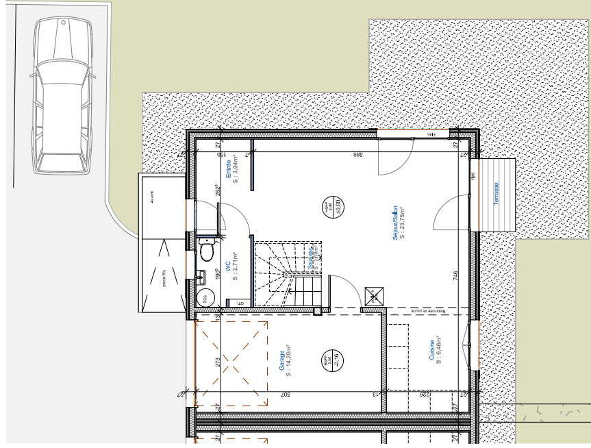
REZ-DE-CHAUSSEE
