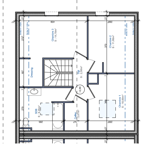
ETAGE
